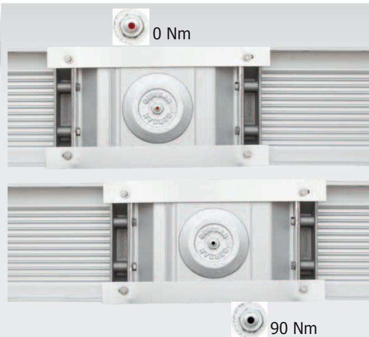
Система контроля степени сжатия соединения
