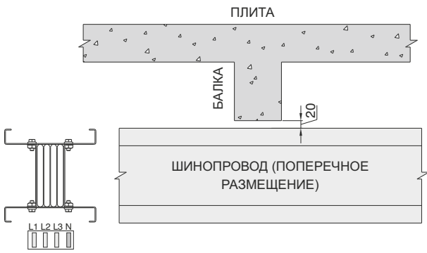
РИСУНОК-7 ПЕРЕСЕЧЕНИЕ ПОД БАЛКОЙ А В ПОПЕРЕЧНОМ РАЗМЕЩЕНИИ
