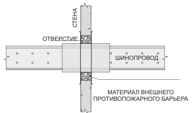
РИСУНОК-5 ПРИМЕР ПЕРЕСЕЧЕНИЯ СТЕНЫ С ПРОТИВОПОЖАРНЫМ БАРЬЕРОМ
