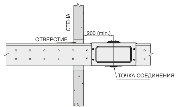
РИСУНОК-6 ПЕРЕСЕЧЕНИЕ СТАНДАРТНОЙ СТЕНЫ
