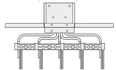
Образец крепления проводников фаз
