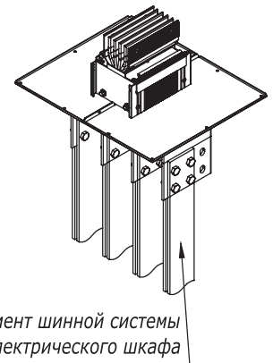
Секция подключения к трансформатору/щиту
