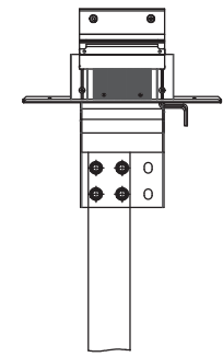
Фрагмент открытой части присоединительной секции шинопровода
